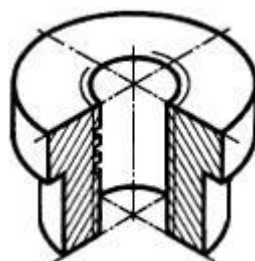
Рисунок А.2 - Нанесение размеров
