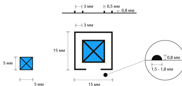
Рисунок 41 - Обозначение лифта на тактильно-визуальной схеме
