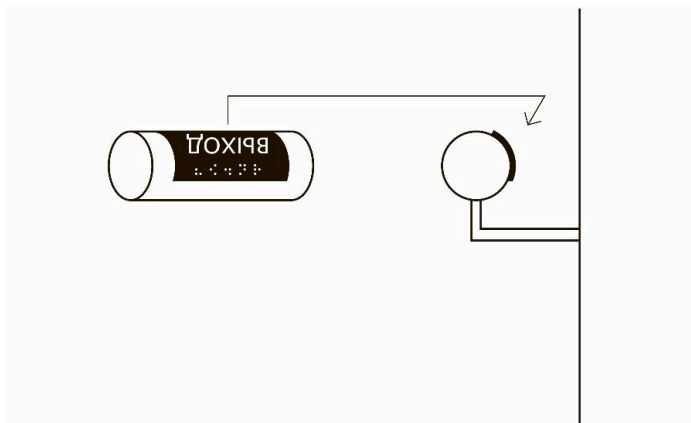
Рисунок 8 - Размещение тактильной информации на поручнях (вид таблички со стороны стены)
