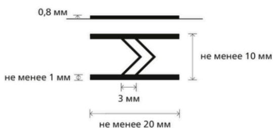
Рисунок 39 - Траволаторы, движущиеся дорожки
