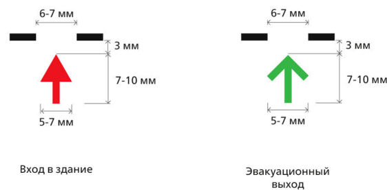
Рисунок 29 - Обозначение входов на объект и эвакуационных выходов
