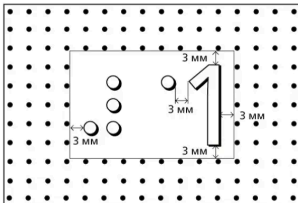
Рисунок 42 - Свободное пространство вокруг меток, встроенных в текстуру
