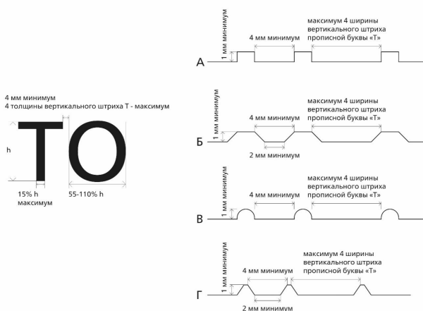
Рисунок 3 Виды рельефов рельефно-линейного шрифта
