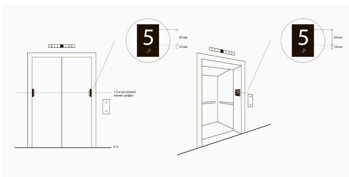
Рисунок 10 — Обозначения номера этажа на боковых поверхностях дверных проемов лифтовой шахты
