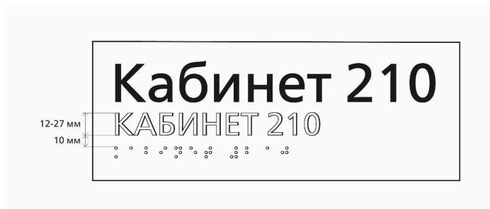
Рисунок 1 Высота рельефно-линейного шрифта при сочетании с плоско-печатным шрифтом (в данном случае рельефные знаки рекомендуется выполнять прозрачными или в цвет подложки)
